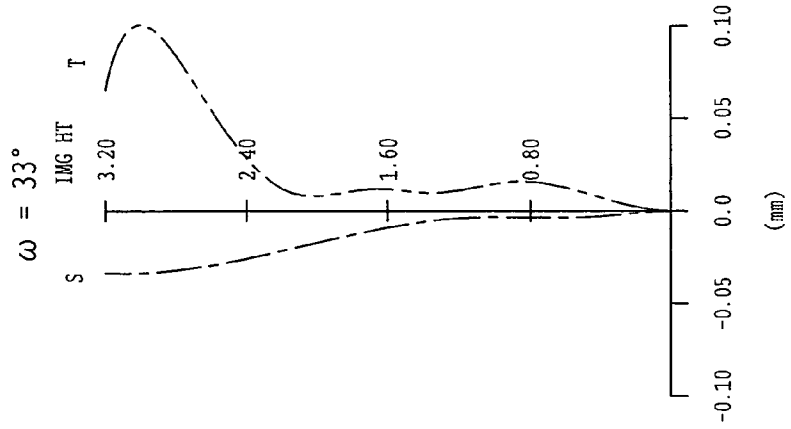
Fig. 8B ASTIGMATISM
